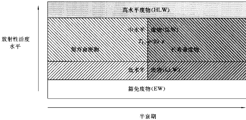
图1 放射性废物分类框架图
